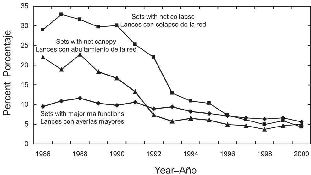
FIGURE 20b. Trends in the malfunctions that can cause dolphin mortalities. FIGURA 20b. Tendencias en averías de las red que pueden causar mortalidad de delfines.
