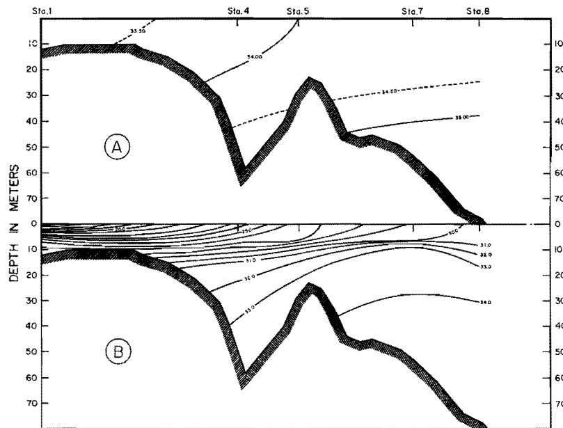
FIGURA 16. Perfiles típicos de la salinidad en el Golfo de Nicoya durante la estación seca (A) y la estación lluviosa (B).
