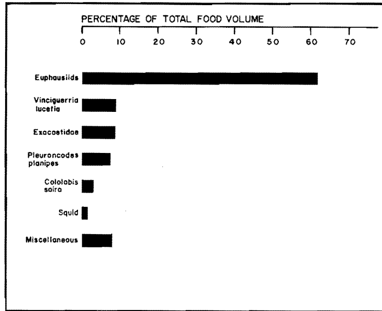
FIGURA 13. Importancia relativa, por volumen, de los principales componentes del alimento del barrilete.
