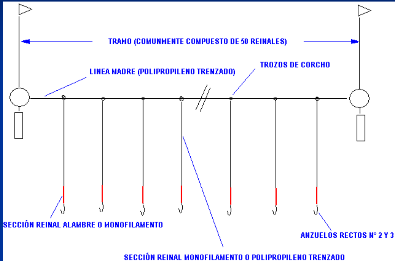
Figura 4 Configuración general del espinel pelágico que opera en la pesquería del dorado
