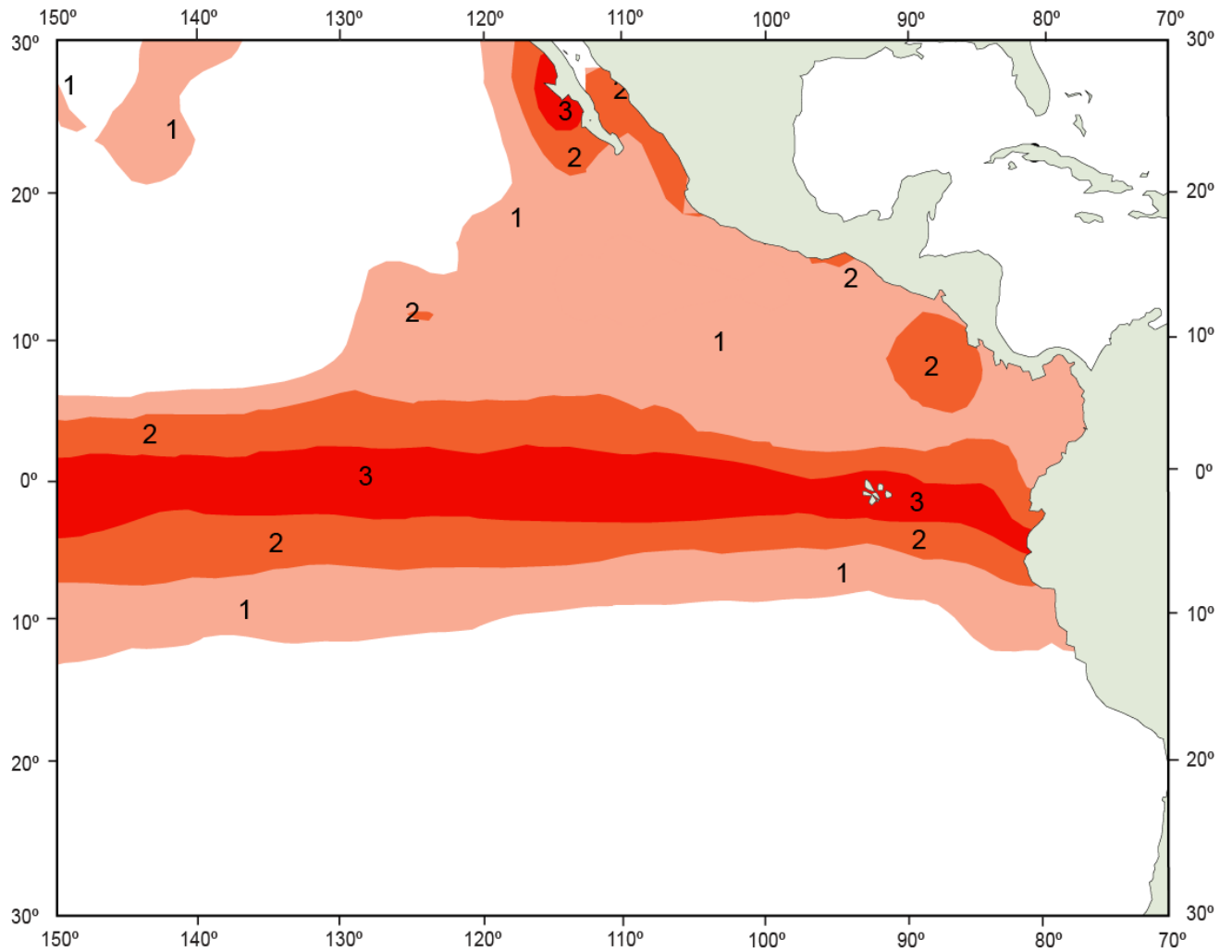
FIGURE 5. Sea-surface temperature (SST) anomalies (departures from long-term normals) for December 2015, based on data from fishing boats and other types of commercial vessels. FIGURA 5. Anomalías (variaciones de los niveles normales a largo plazo) de la temperatura superficial del mar (TSM) en diciembre de 2015, basadas en datos tomados por barcos pesqueros y otros buques comerciales.
