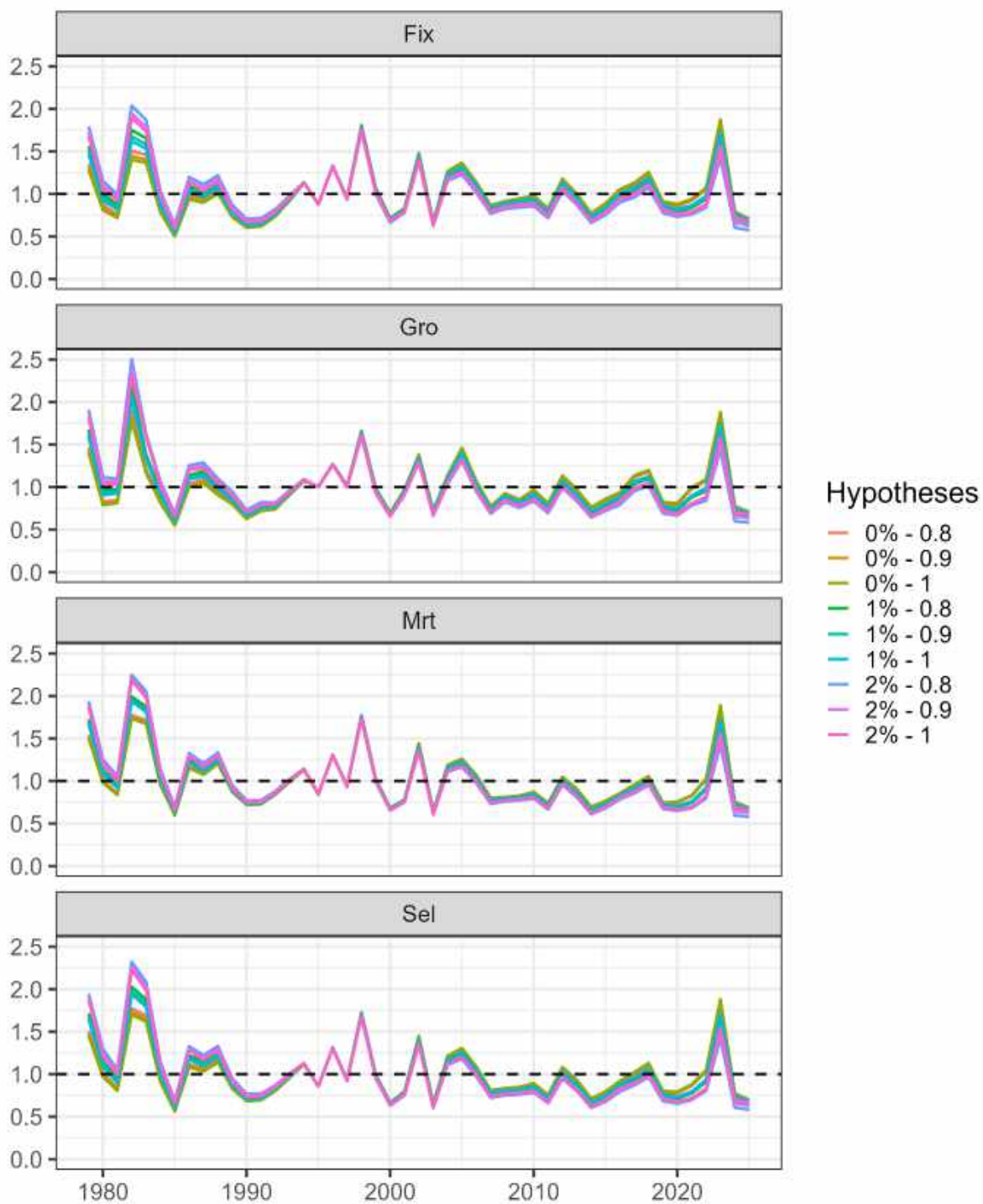
FIGURE D-2. Comparison of estimated relative annual recruitment of bigeye tuna between 1979 and 2025. FIGURA D-2. Comparación del reclutamiento anual relativo estimado del atún patudo entre 1979 y 2025.
