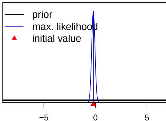
SizeSpline_Val_10_F18-DEL_C(18)
