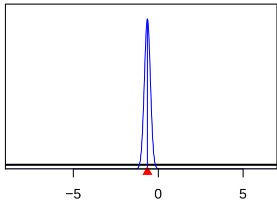
SizeSpline_Val_2_F1-OBJ_N-Q14(1)
