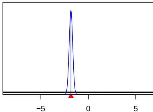
SizeSpline_Val_2_F11-NOA_N(11)
