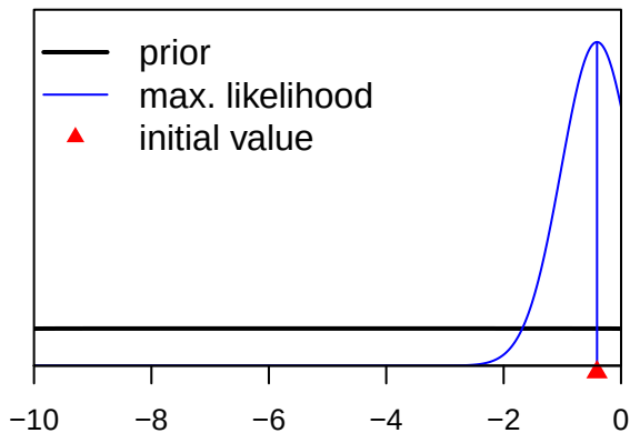
SizeSpline_Val_2_F1-OBJ_N-Q14(1)
