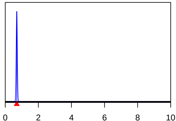
SizeSpline_GradHi_S4-PS_late_VAST(44)
