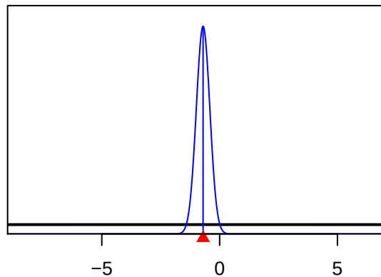
SizeSpline_Val_4_S4-PS_late_VAST(44)
