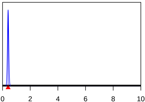
SizeSpline_GradLo_F15-DEL_N(15)
