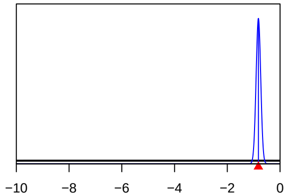
SizeSpline_GradHi_S4-PS_late_VAST(44)
